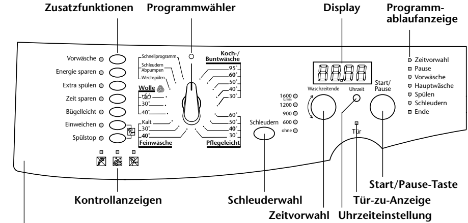
Bedienblende Waschmittelschublade
